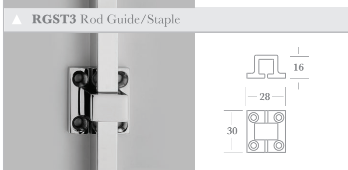
▲ RG3 Rod Guide
