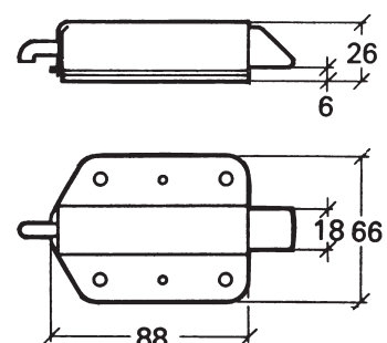
End bolt 1185
